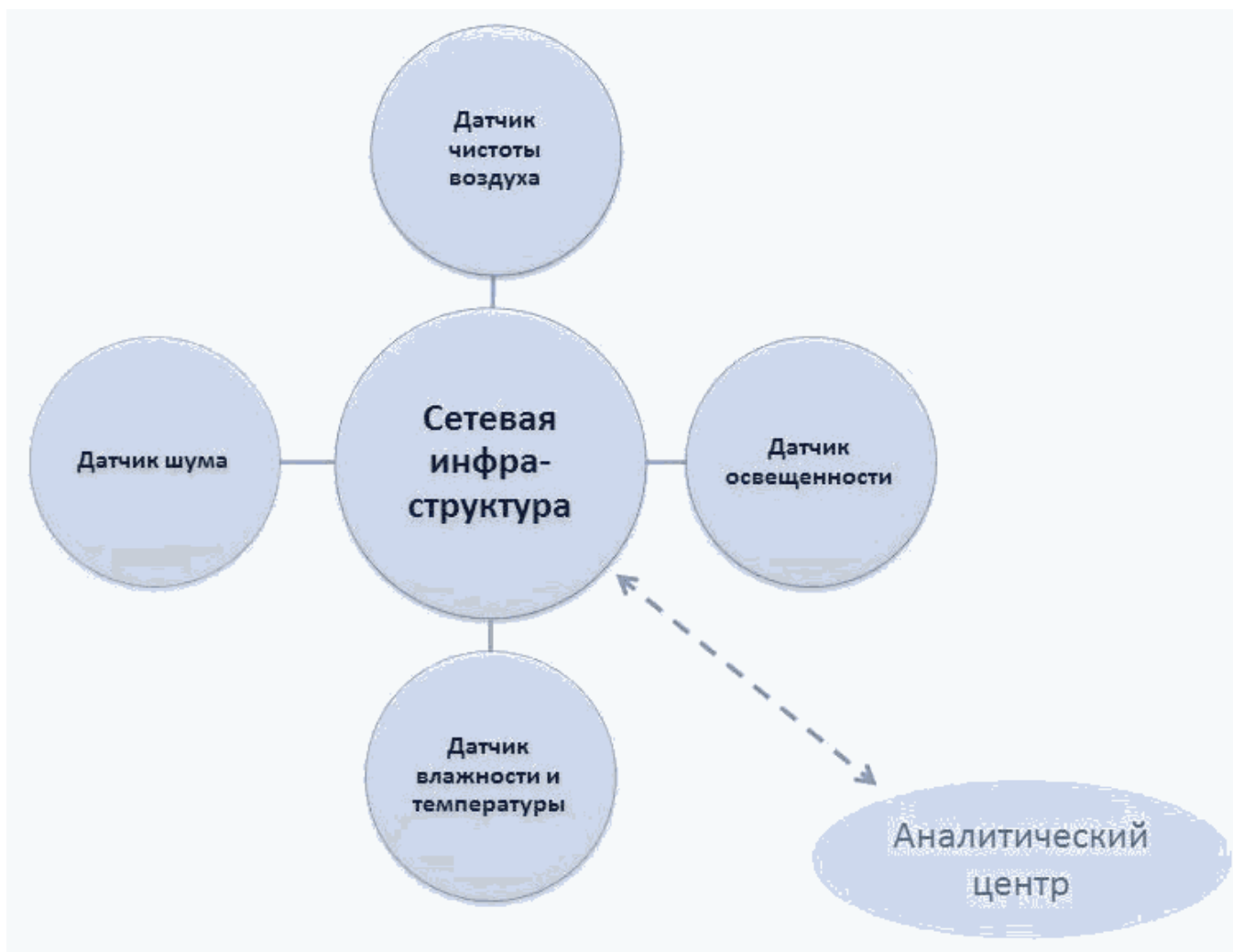
Рис. 14. Организация городской системы фиксации вредных выбросов
